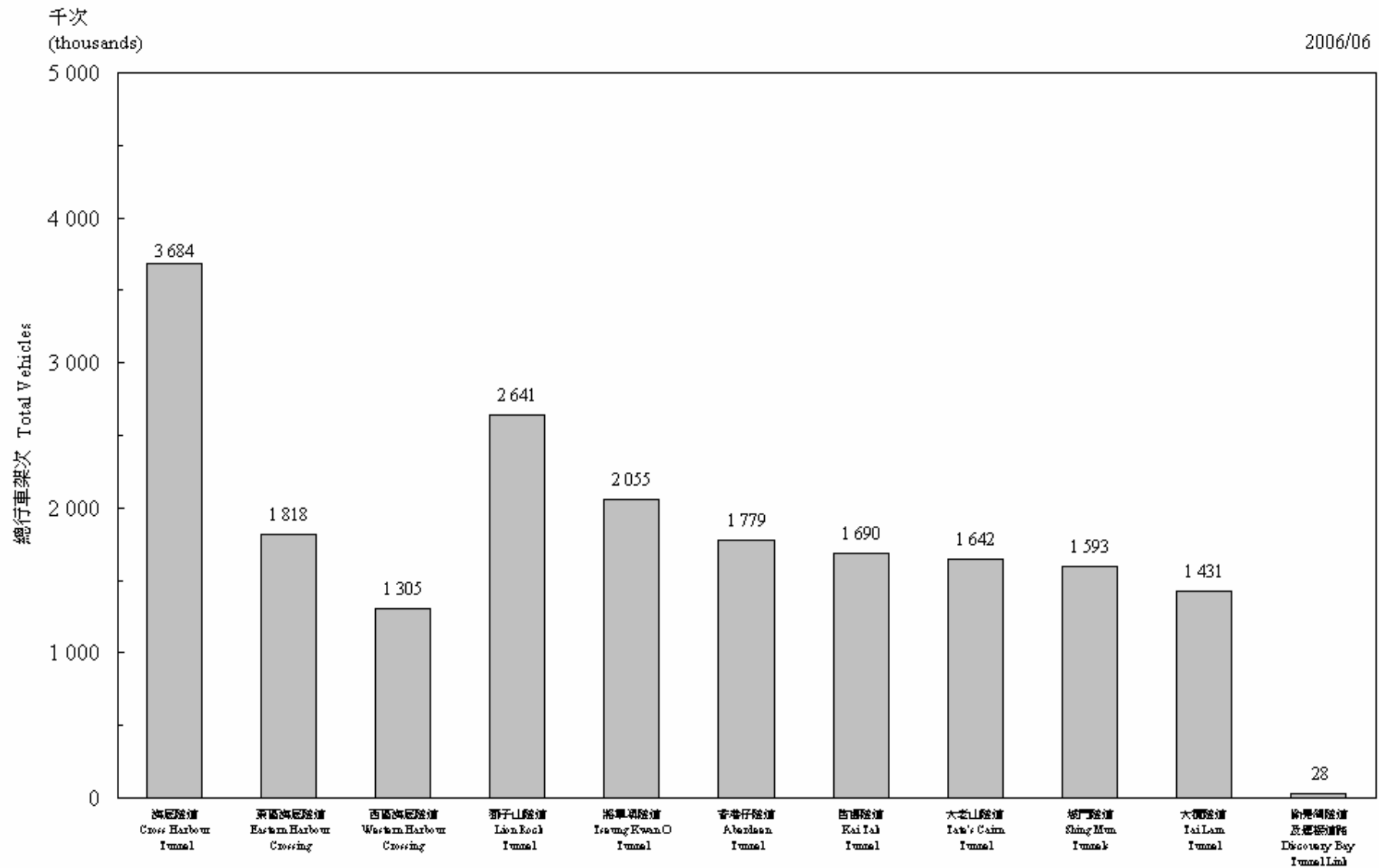
圖 3.1 - 隧道交通流量 (2006年6月) Chart 3.1 - Vehicular Traffic Through Tunnels (June 2006)
