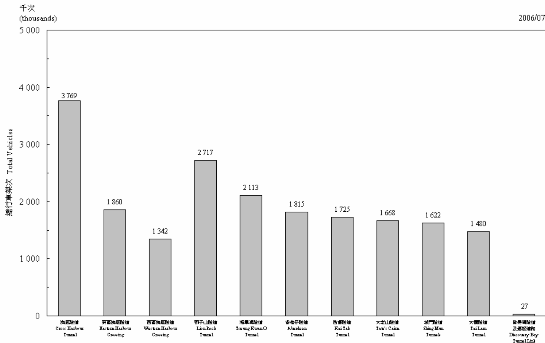
圖 3.1 - 隧道交通流量 (2006年7月) Chart 3.1 - Vehicular Traffic Through Tunnels (July 2006)
