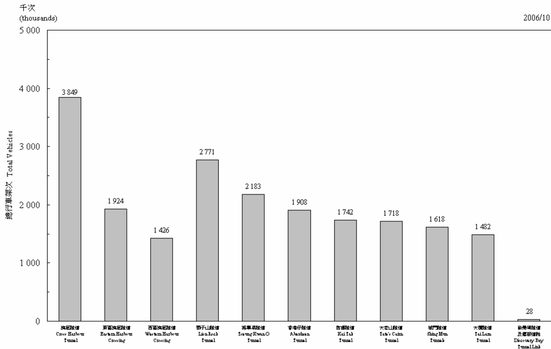
圖 3.1 - 隧道交通流量 (2006年10月) Chart 3.1 - Vehicular Traffic Through Tunnels (October 2006)
