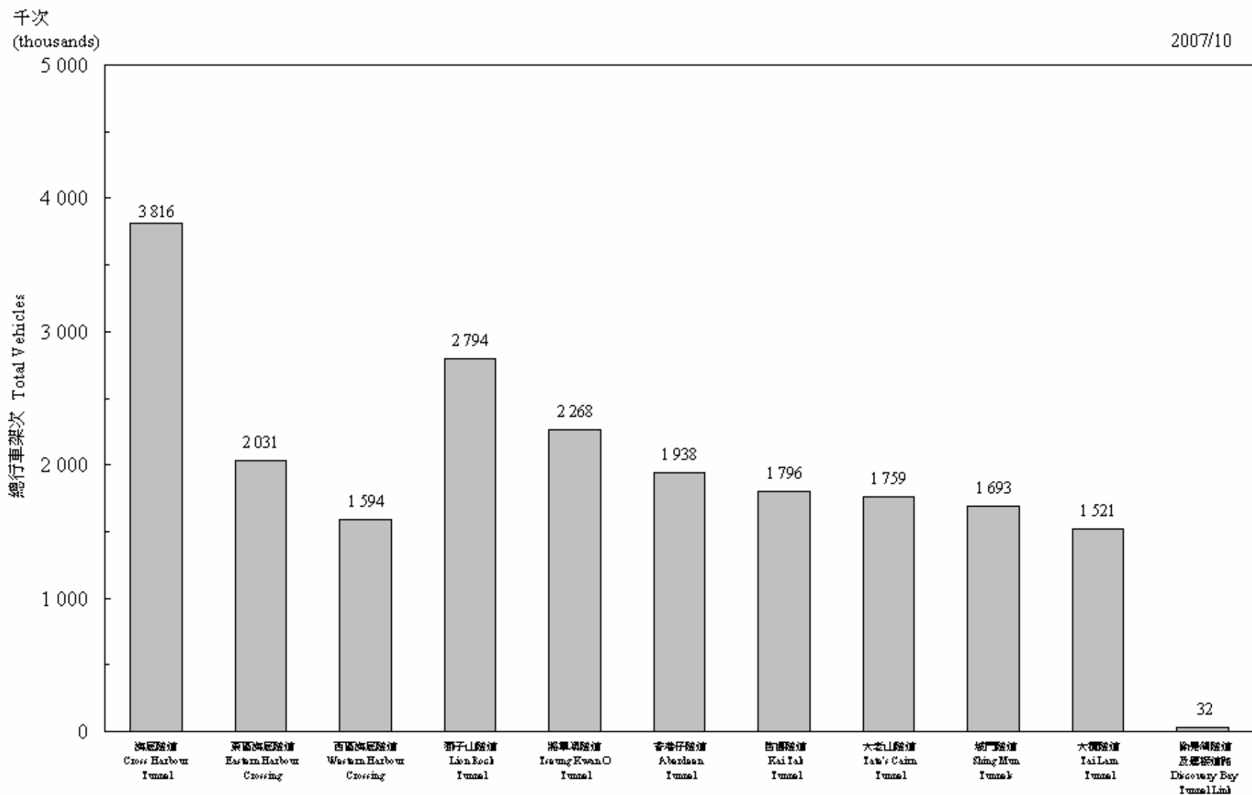
圖 3.1 - 隧道交通流量 (2007年10月) Chart 3.1 - Vehicular Traffic Through Tunnels (October 2007)
