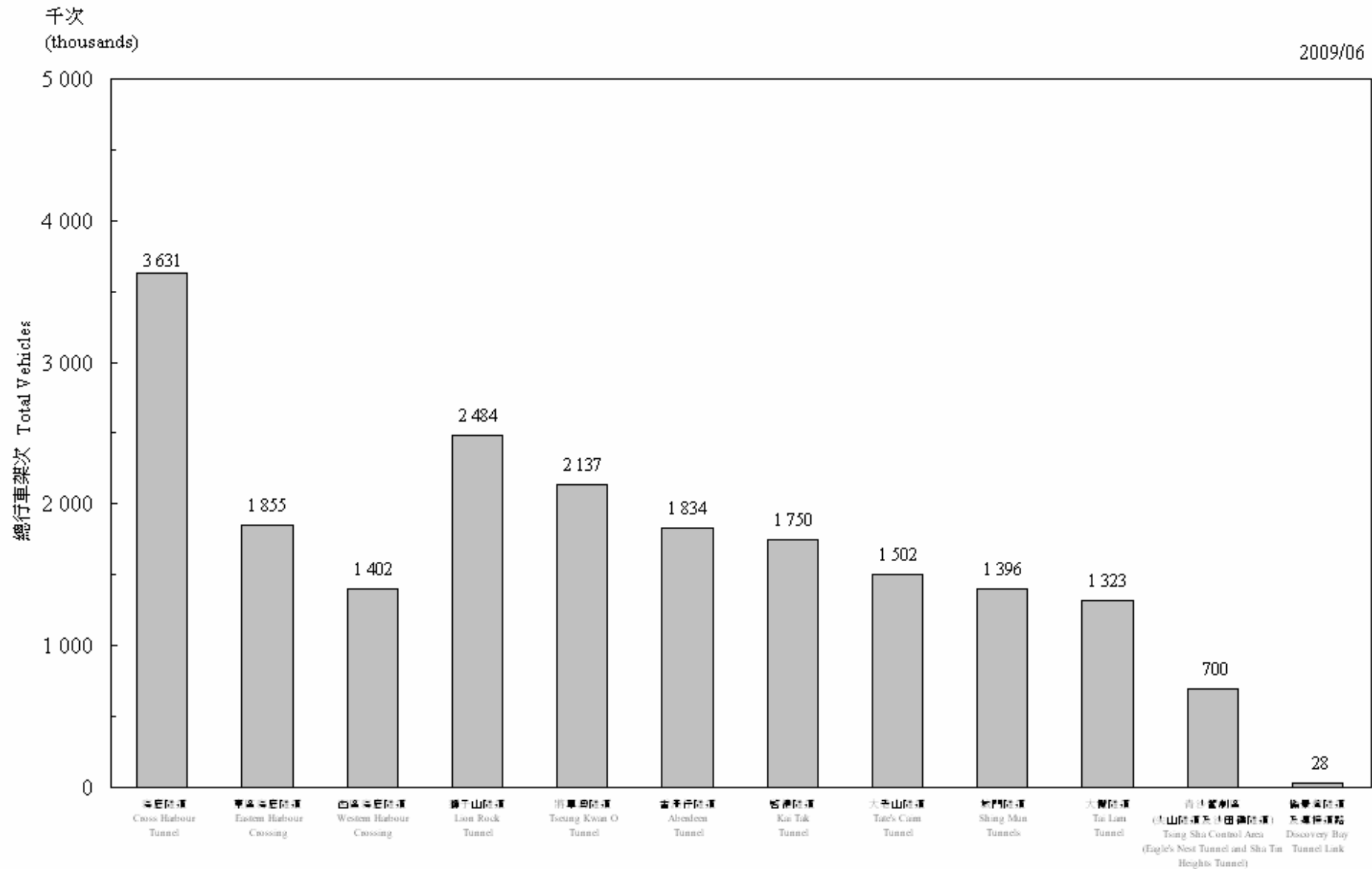
圖 3.1 - 隧道交通流量 (2009年6月) Chart 3.1 - Vehicular Traffic Through Tunnels (June 2009)
