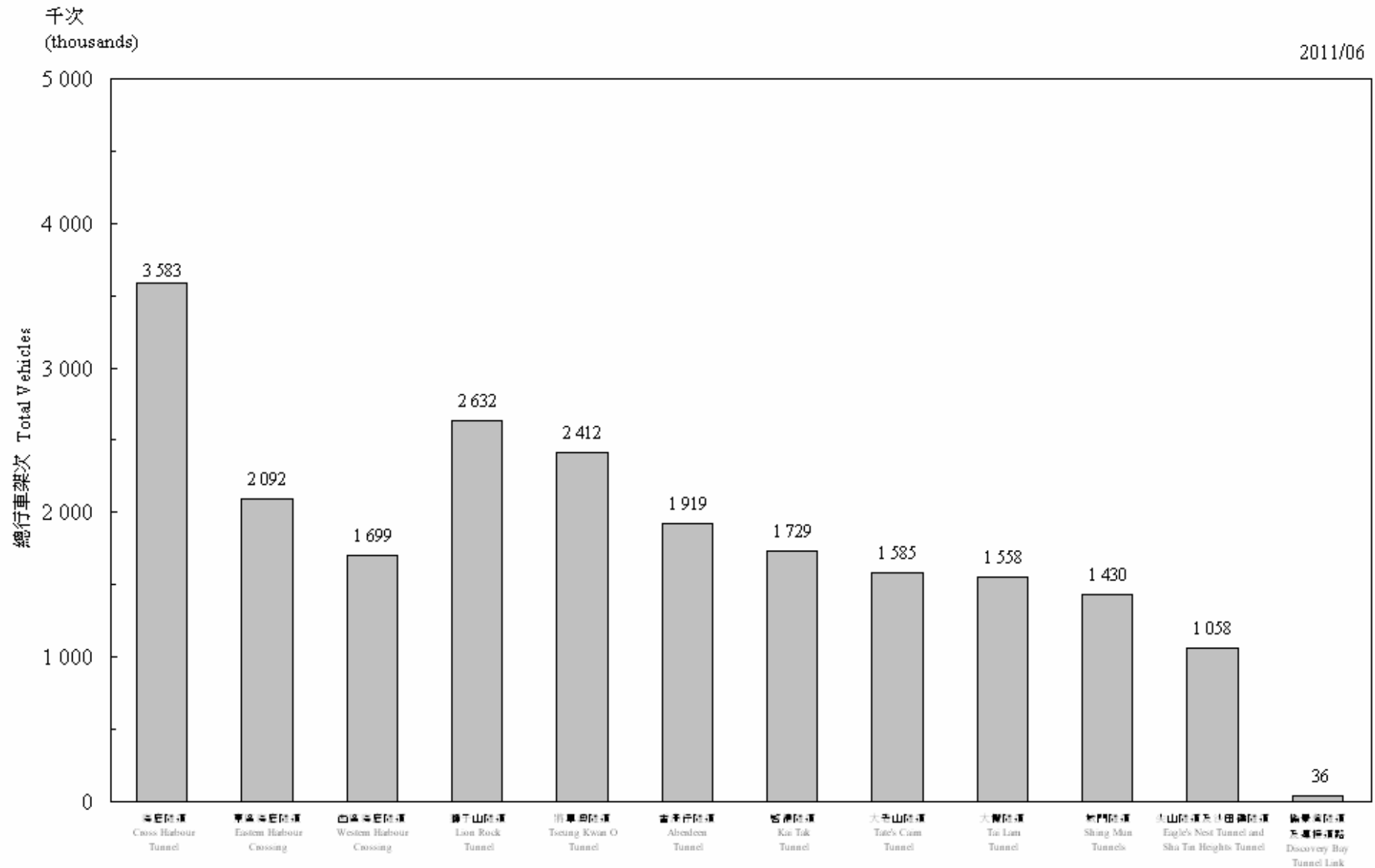
圖 3.1 - 隧道汽車流量 (二零一一年六月) Chart 3.1 - Vehicular Flow Through Tunnels (June 2011)
