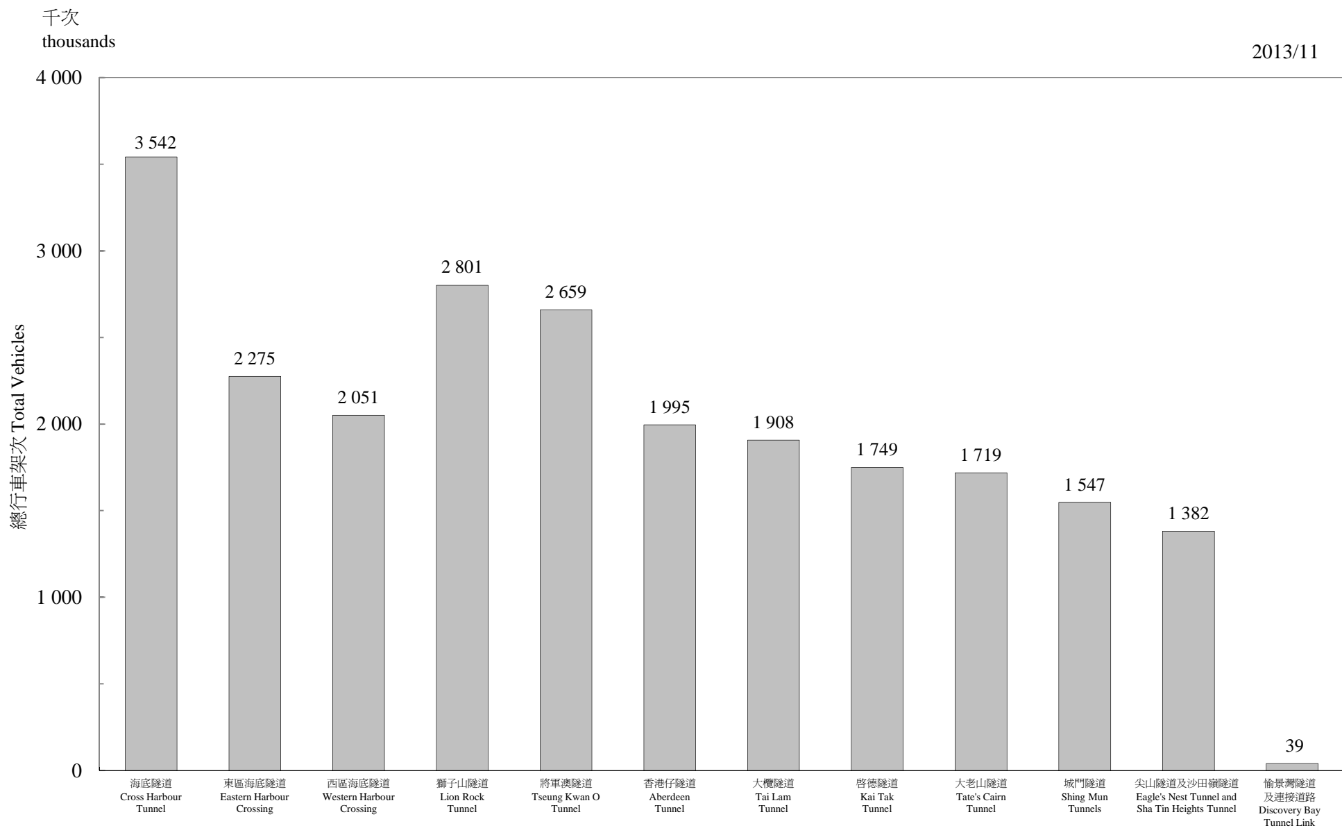
圖 3.1 - 隧道汽車流量 (二零一三年十一月) Chart 3.1 - Vehicular Flow Through Tunnels (November 2013)
