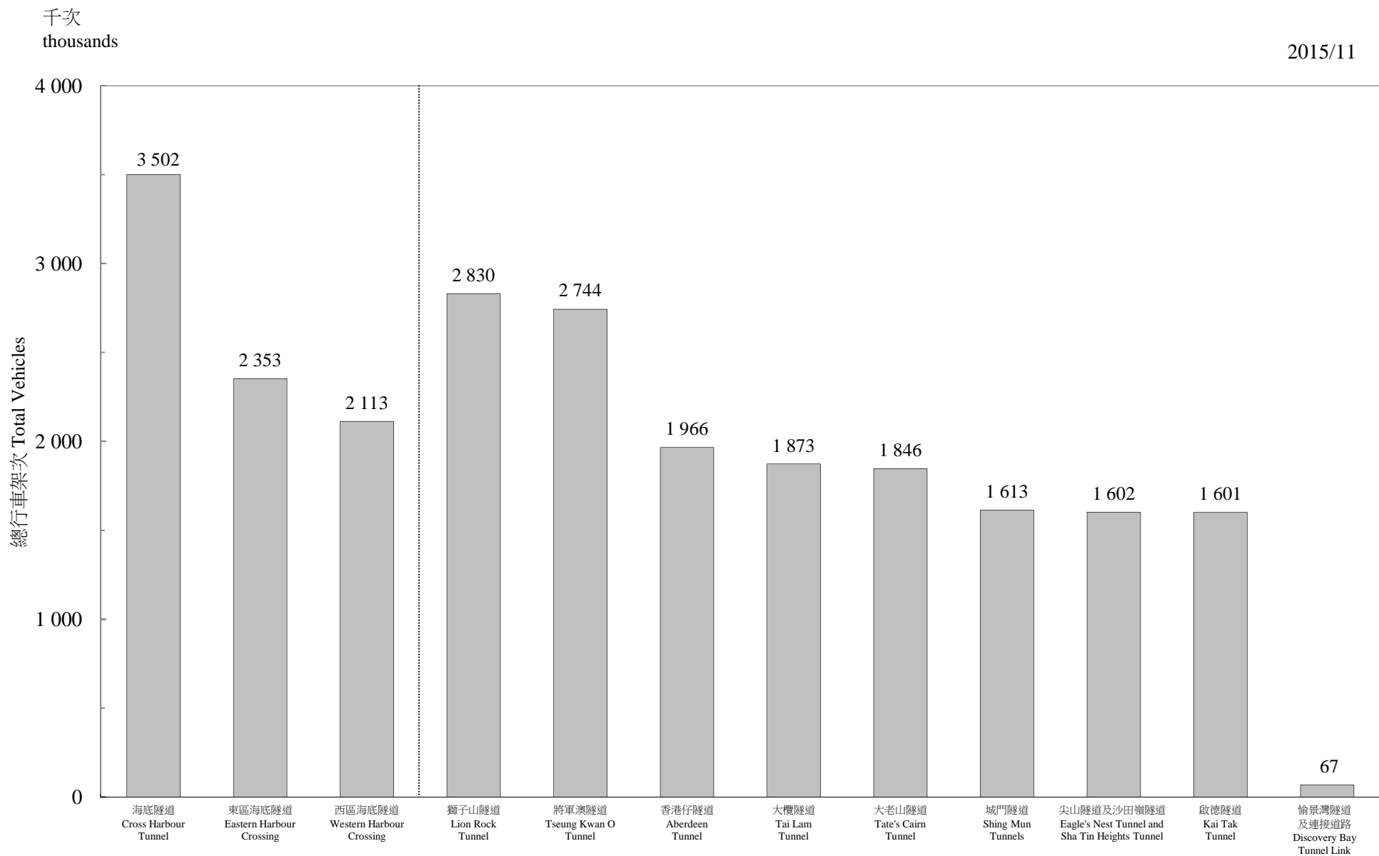
圖 3.1 - 隧道汽車流量 (二零一五年十一月) Chart 3.1 - Vehicular Flow Through Tunnels (November 2015)
