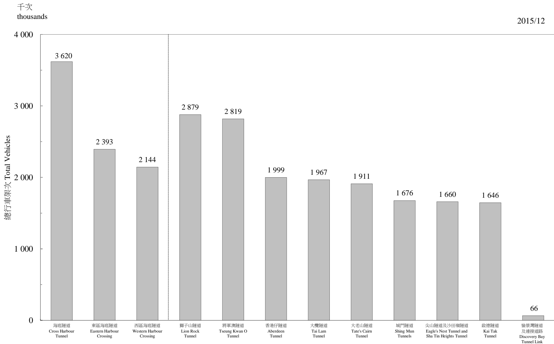
圖 3.1 - 隧道汽車流量 (二零一五年十二月) Chart 3.1 - Vehicular Flow Through Tunnels (December 2015)
