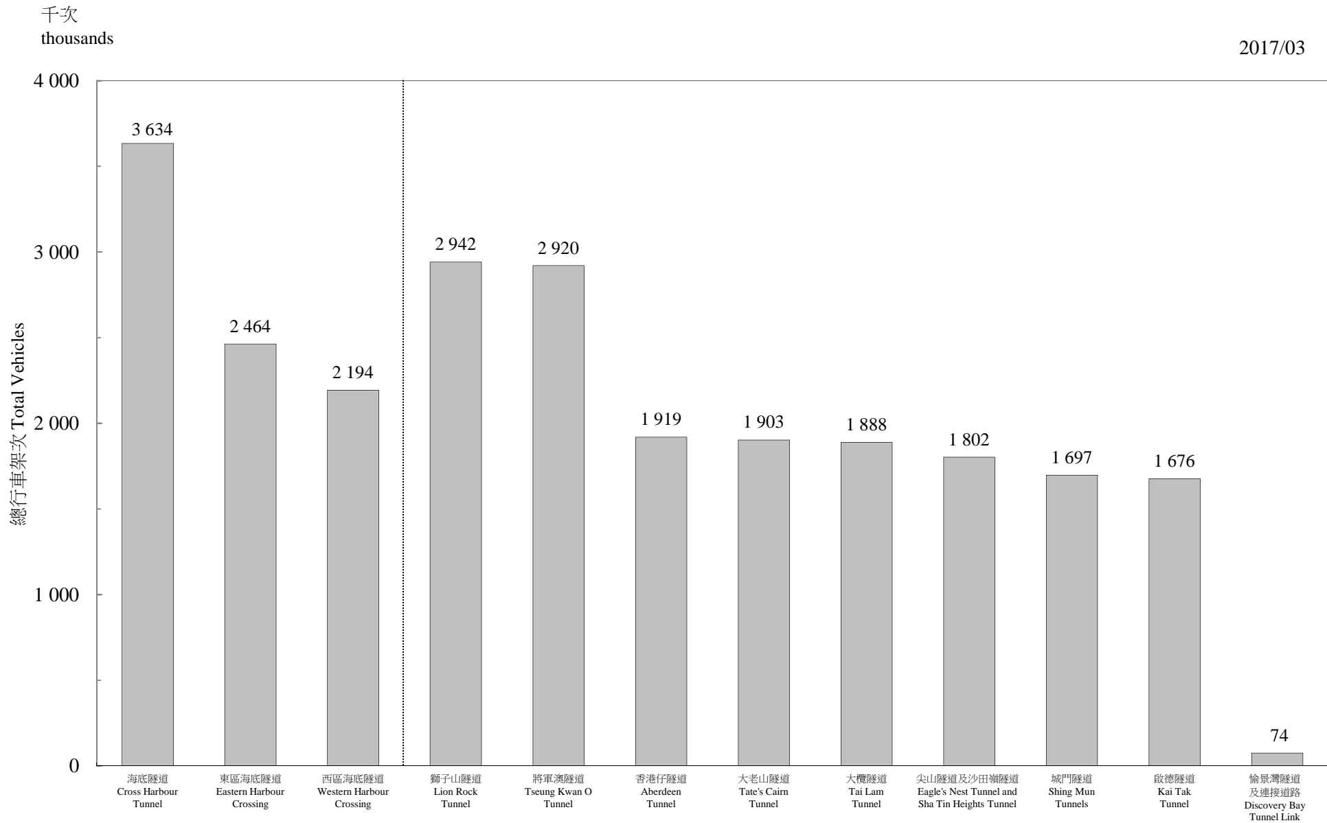
圖 3.1 - 隧道汽車流量 (二零一七年三月) Chart 3.1 - Vehicular Flow Through Tunnels (March 2017)
