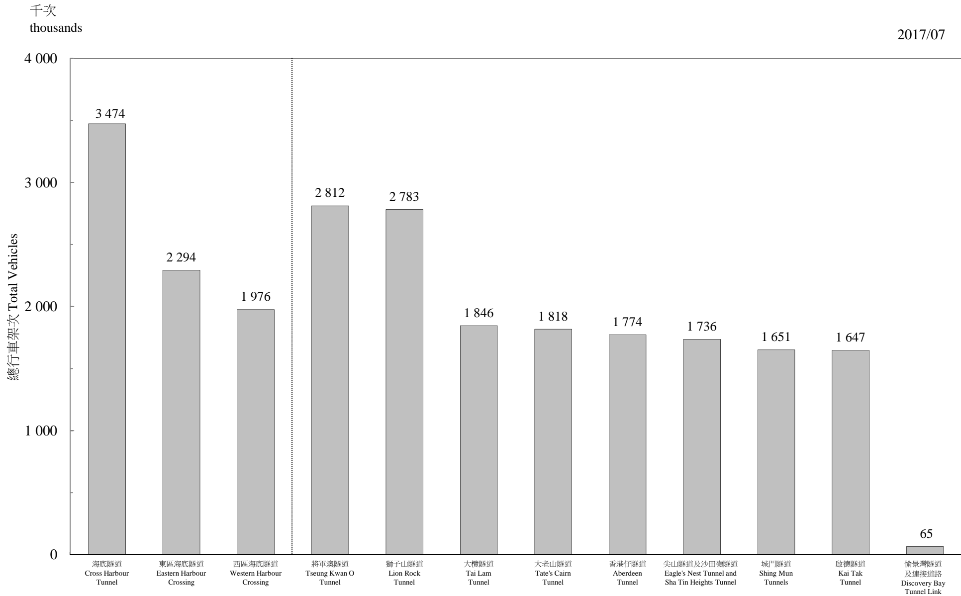
圖 3.1 - 隧道汽車流量 (二零一七年七月) Chart 3.1 - Vehicular Flow Through Tunnels (July 2017)
