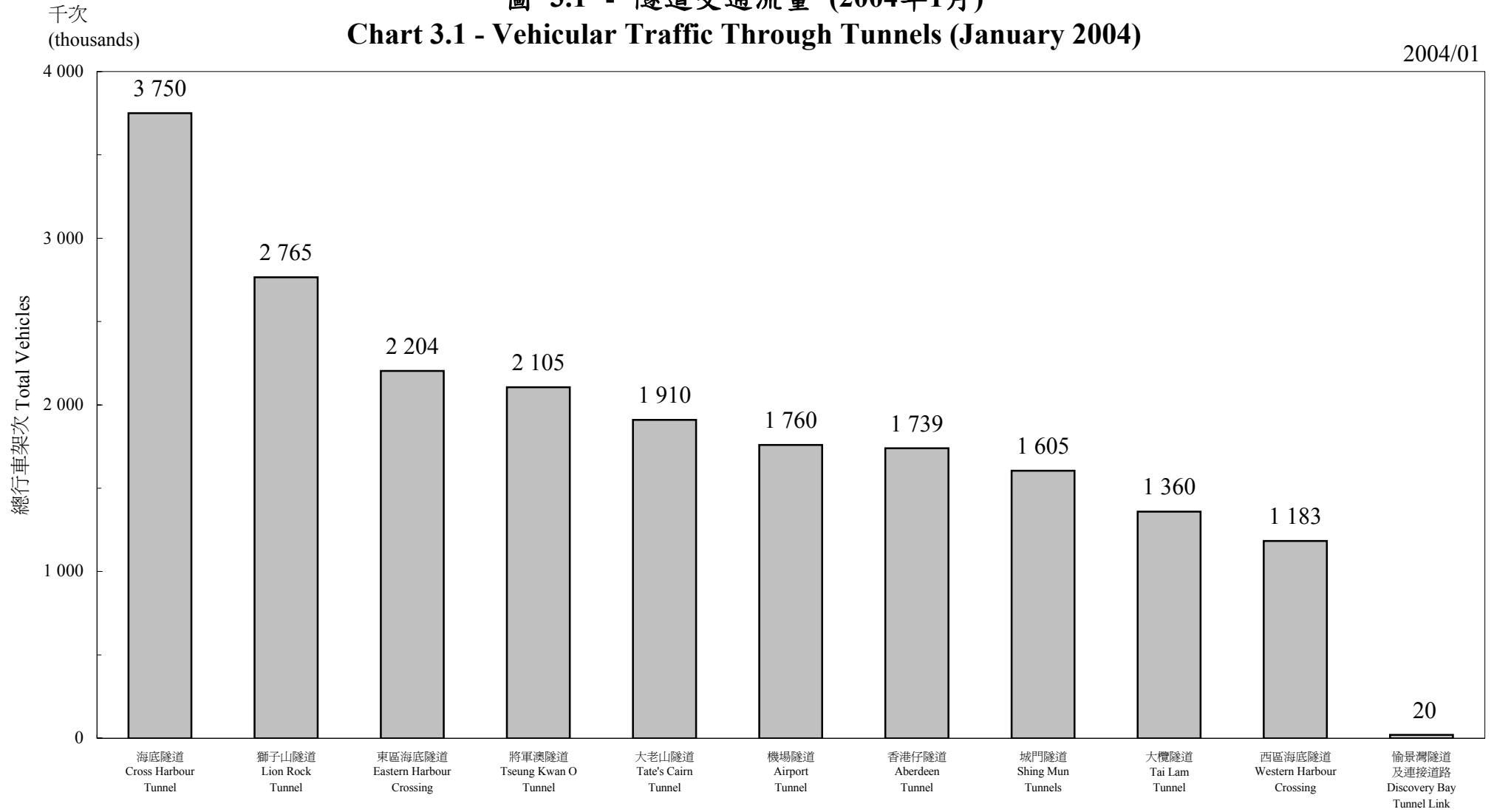
圖 3.1 - 隧道交通流量 (2004年1月)
